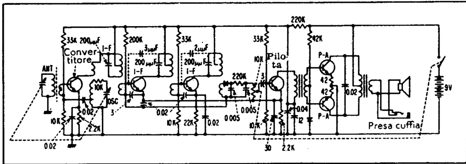
SCHEMA ELETTRICO DEL RADIORICEVITORE « SONY TR-63 » DELLA TOKYO TSUSHIN KOGYO, Ltd.
